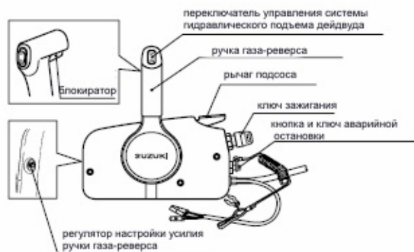
МАШИНКА ГАЗА-РЕВЕРСА
