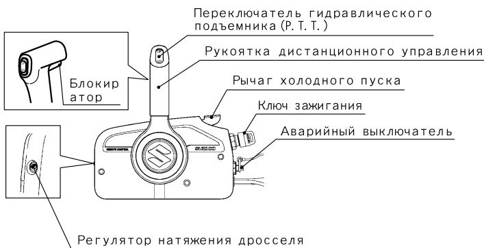
УЗЕЛ ДИСТАНЦИОННОГО УПРАВЛЕНИЯ
